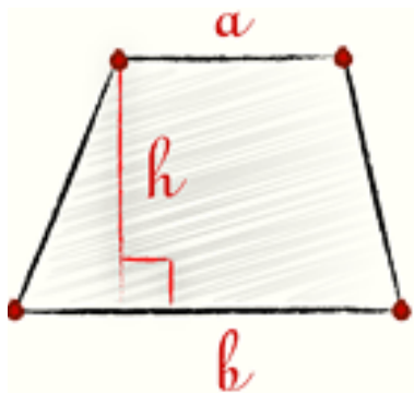
Рис. 1 Трапеция
